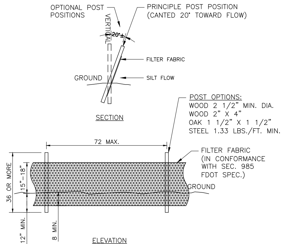
3 F.D.O.T. TYPE E-1 SILT FENCE SCALE: N.T.S.
